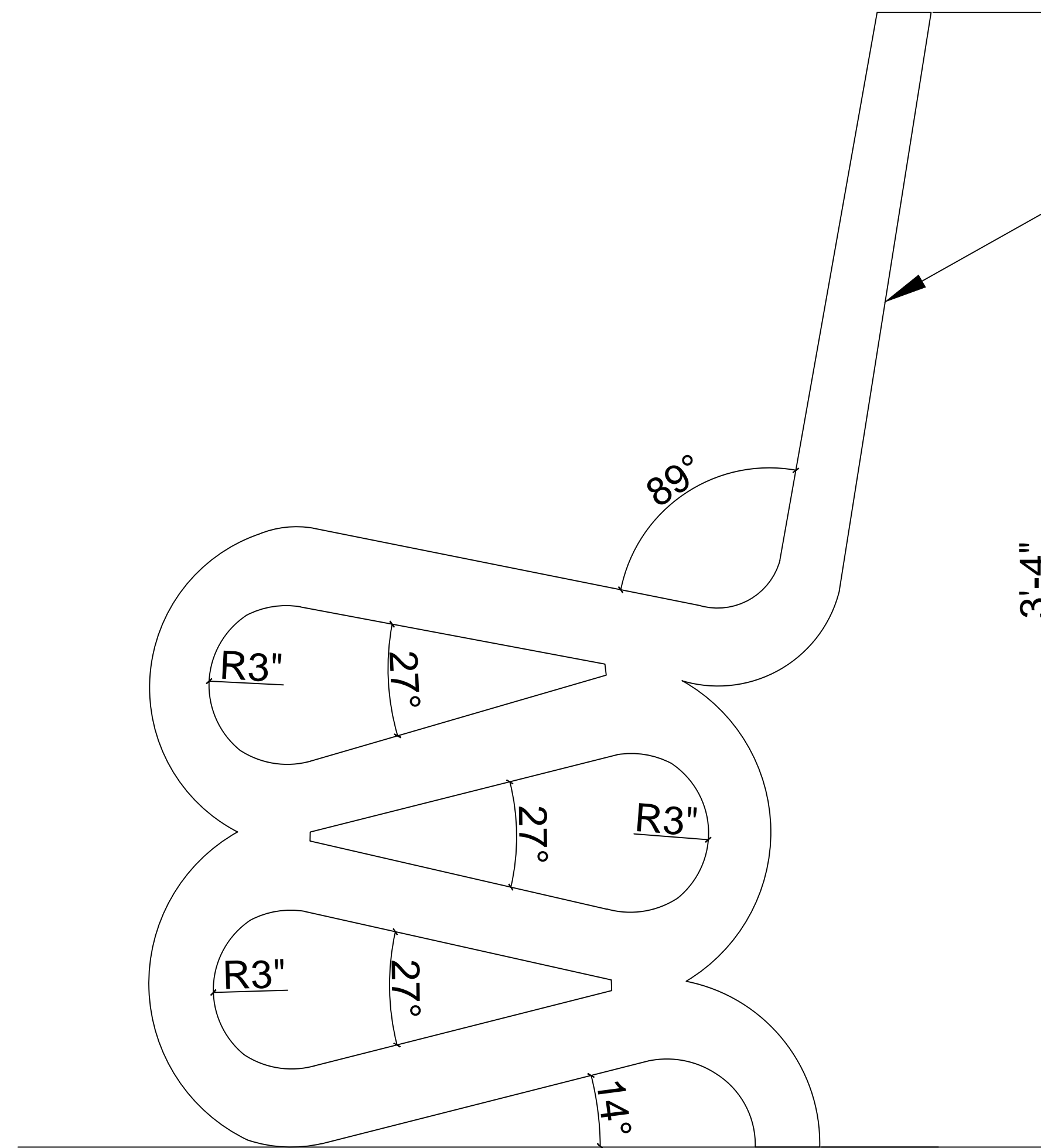
SECTION SCALE: 3" = 1'-0"
