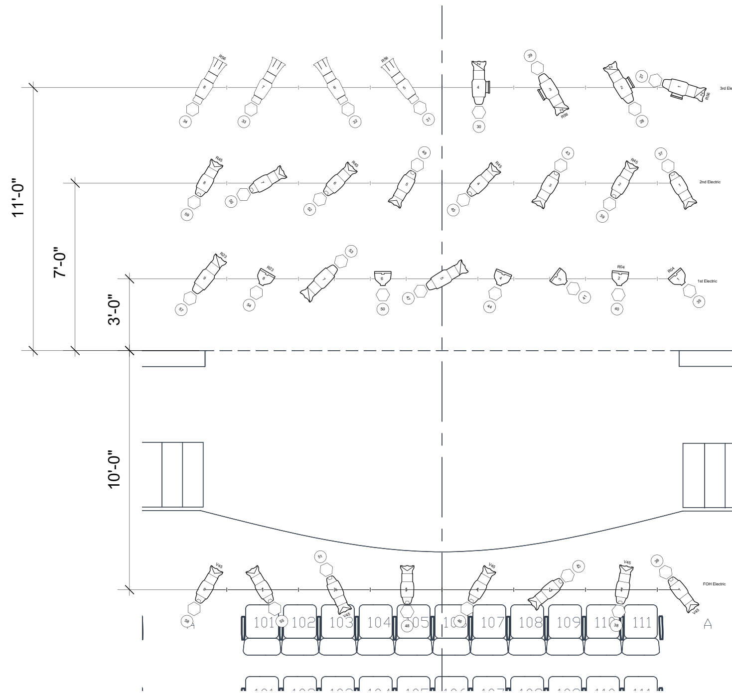
1 LP Plot Scale: 1/4" = 1'-0"
