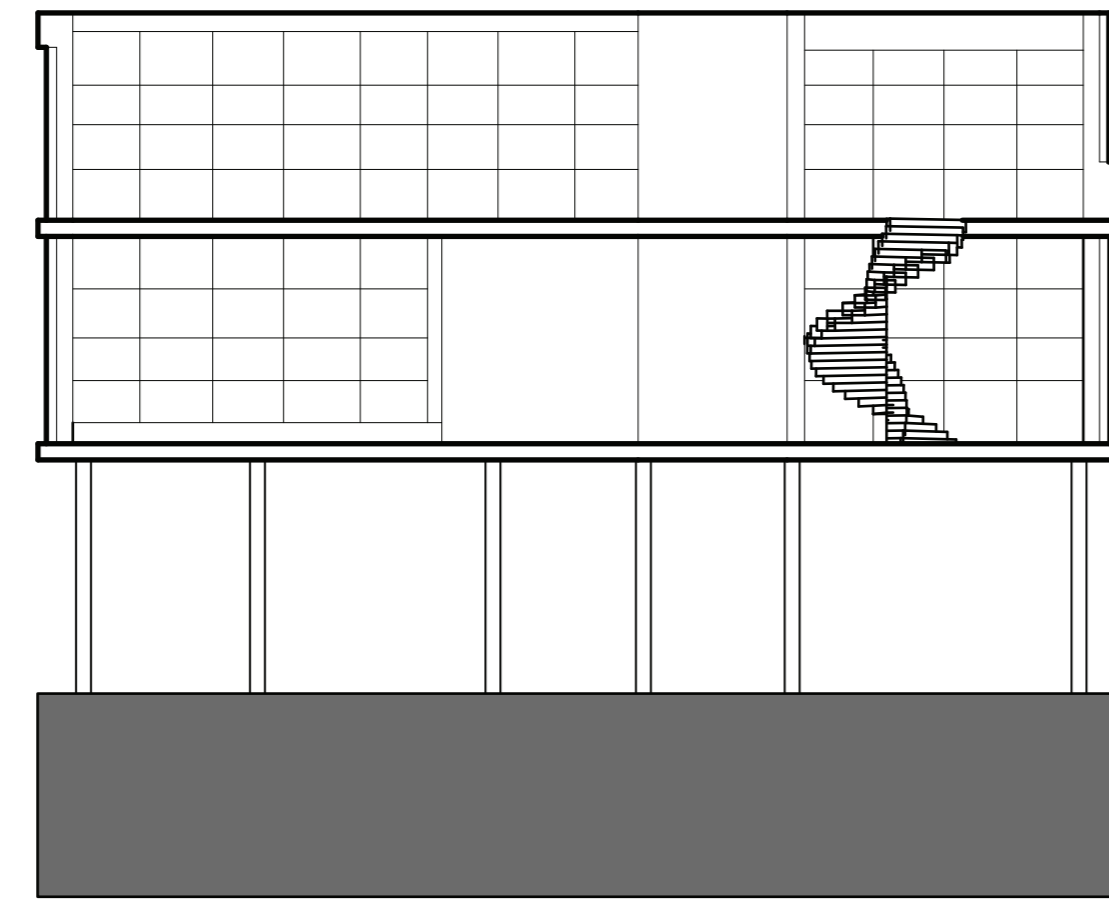
Longitudinal Section
