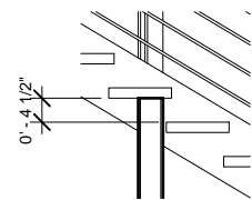
⑧ Riser 2 1/2" = 1'-0"
