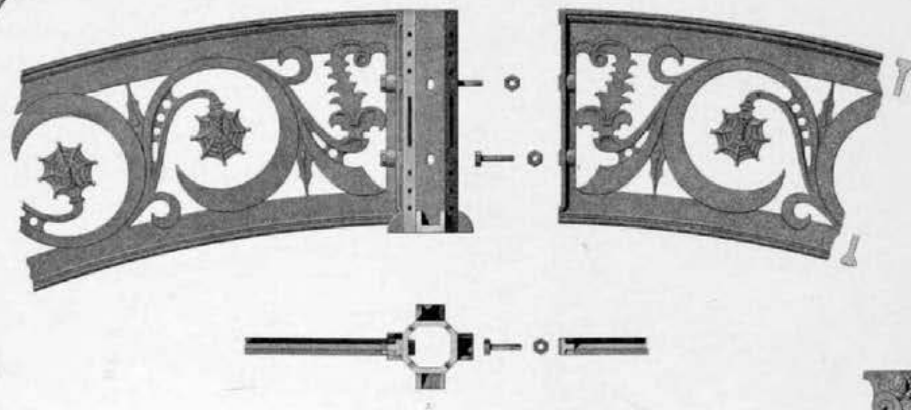
Fig. 3. Clé et milieu des grands arcs.
