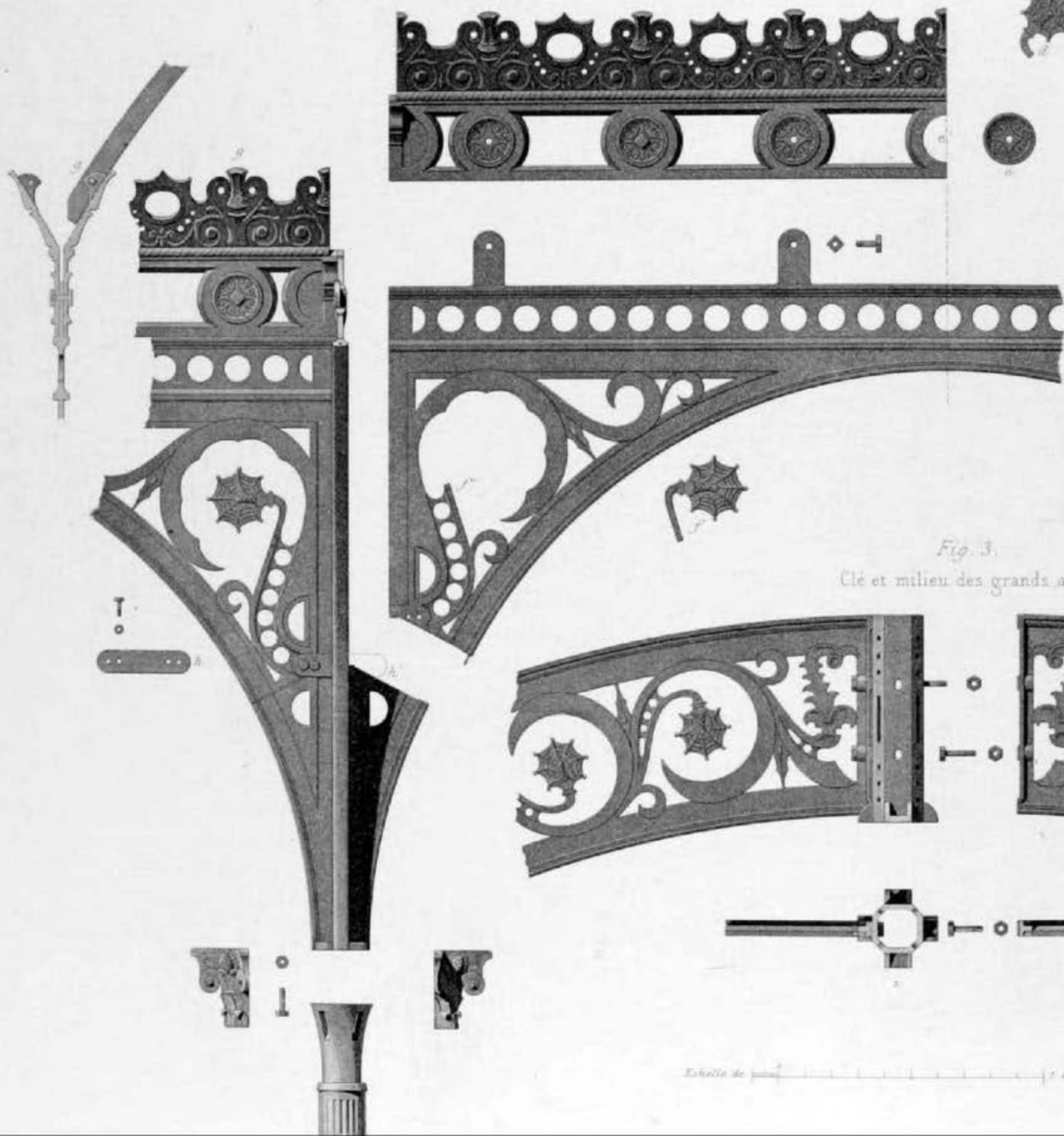
Fig. 2. Petits arcs et galerie de couronnement.
