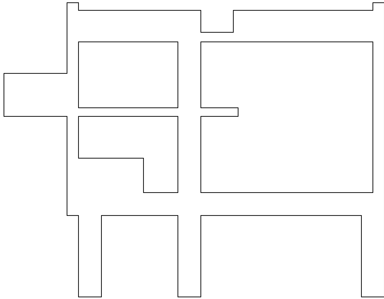
(A-502) PIER B-1,2,3 SCALE 1/4"=1'-0"
